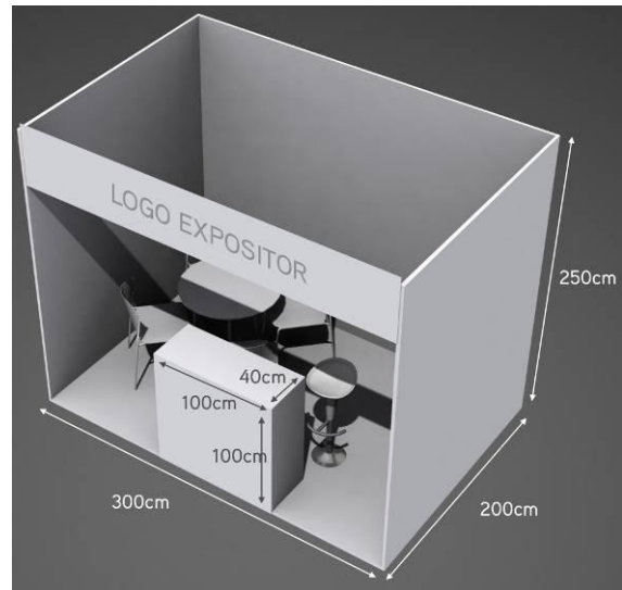
Estand de expositor. 3x2m de planta y 2,5m de altura
